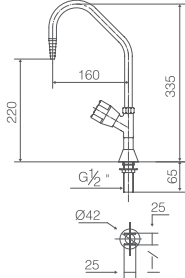
WJH0911 单联化验水咀 Single Assay Faucet
