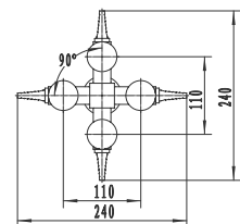
FQ4401A 四开立式供气咀 Four Way Erect Gas Tap
