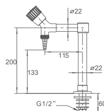
F1122 单联化验水咀 Single Assay Faucet
