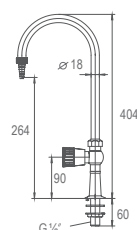
F1101 单联化验水咀 Single Assay Faucet
