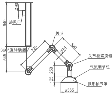
WJH0607-3L 万向顶式抽气罩（三节，铝合金） Aluminium Alloy 3 Joints Fume Extractor
