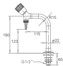
F1112 单联化验水咀 Single Assay Faucet
