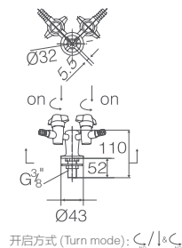
WJH0802AB1 双开立式供气咀（安全弹扣开启） Two Way Erect Gas Valve(Safety Press-turn Open)
